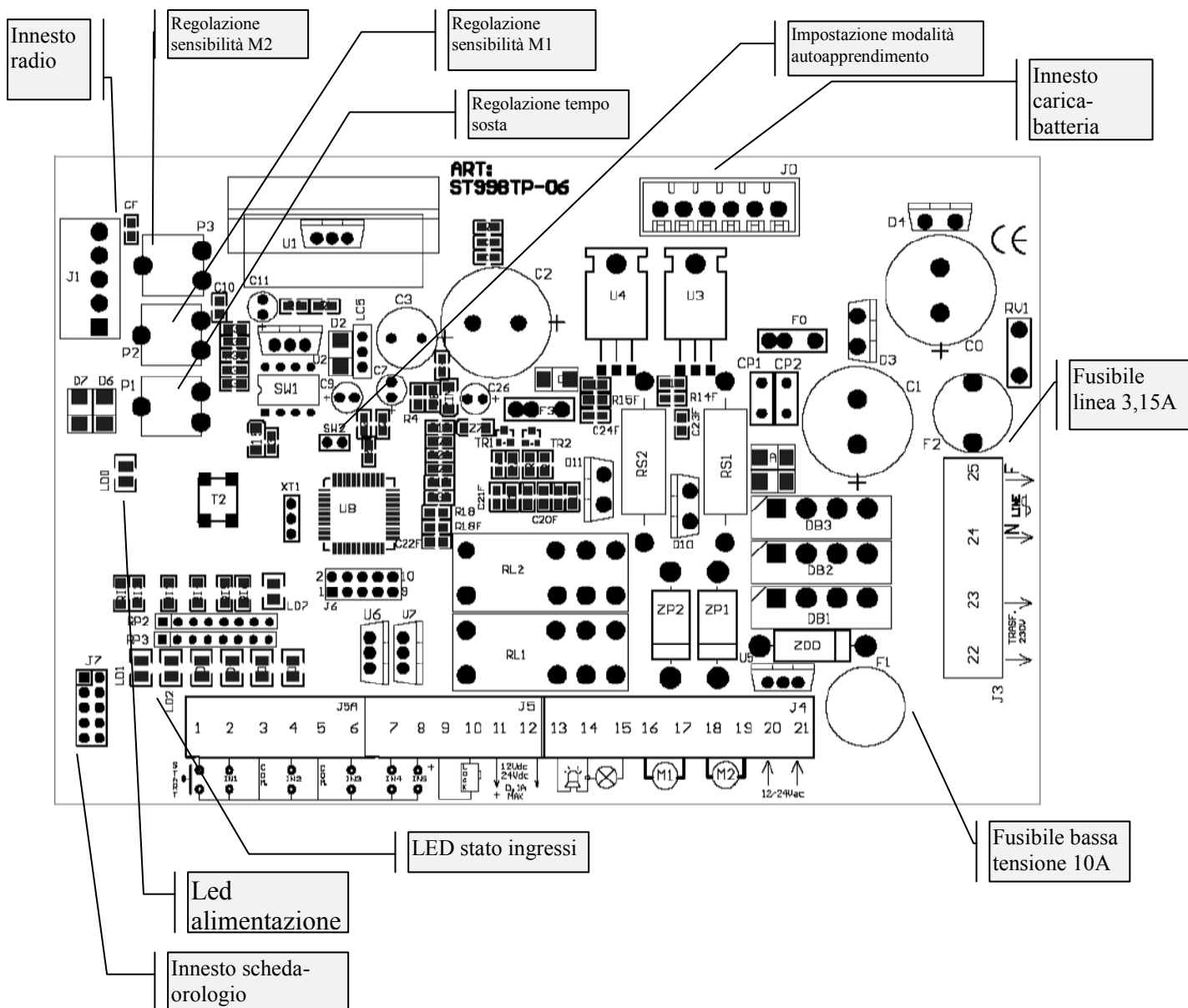
Figura 1 : Lay Out Centralina ST99BTP-06
